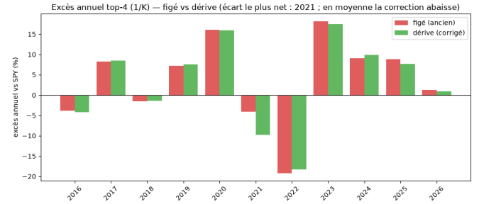
FIGURE 3 – Excès annuel top-4 (1/ K ) : combinaison figée vs corrigée (écart le plus net en 2021).
